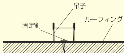
■断面詳細図
