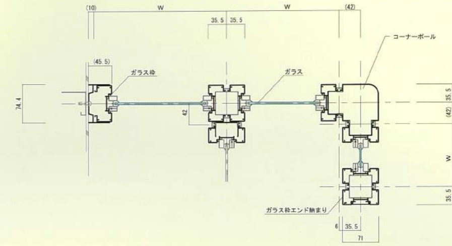
ガラス 横断面図
