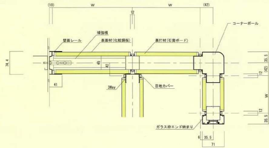
パネル 横断面図
